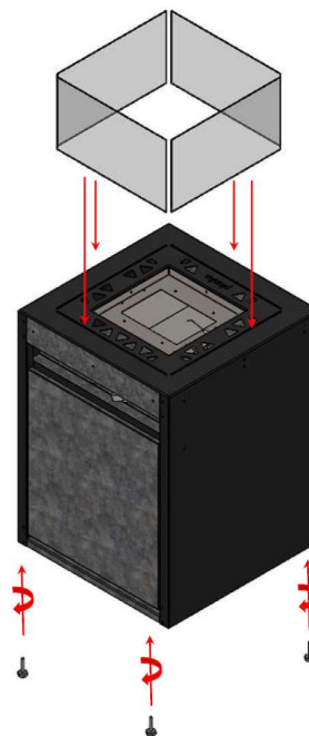
Abbildung 3 – Montage der Glasscheiben
